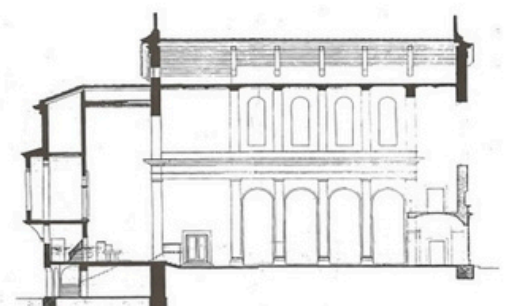
Façanes i secció longitudinal del projecte de Ramon Aragó Cabanes. © Josep Barahona.
